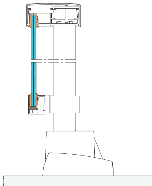
Coupe verticale
