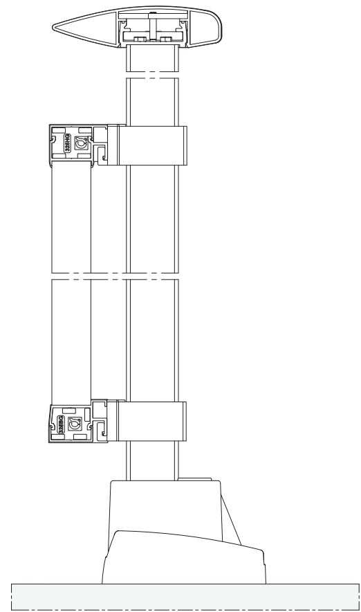
Coupe verticale
